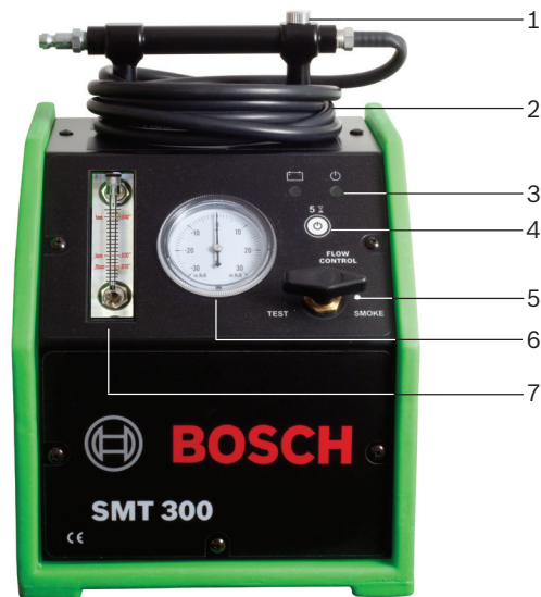
插图 1: SMT 300 正视图
