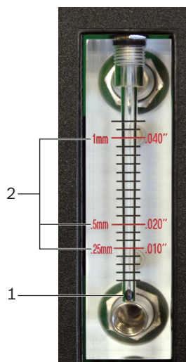
Abb. 3: Übersicht Durchflussmesser
