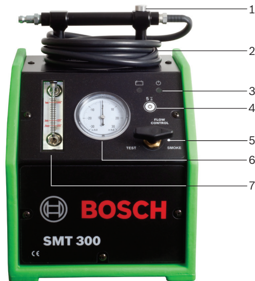
Abb. 1: Frontansicht SMT 300
